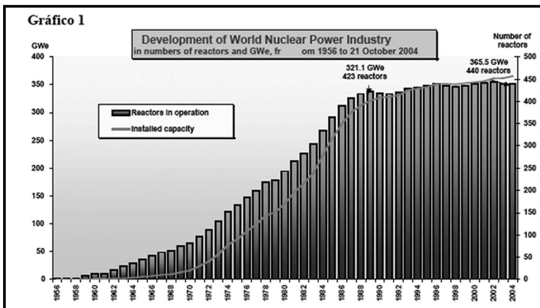
Nombre de reactors i potència instal·lada al món Font: World Nuclear Industry Status Report 2004
